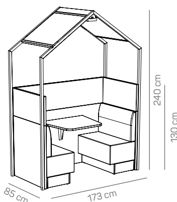
Treinzit + lage opzetwanden + huisje
