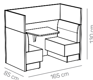
Treinzit + lage opzetwanden
